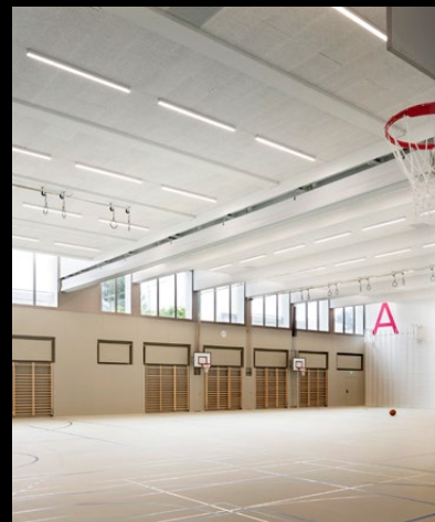
Turnhalle: Langfeld-Aufbauleuchte „Inline M“ in Standardversion mit Schutzvorrichtung.
