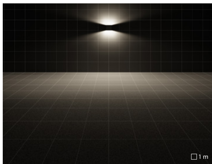
MIMIK 50 B | CP/T2 optique pour velos et pietons type 2
