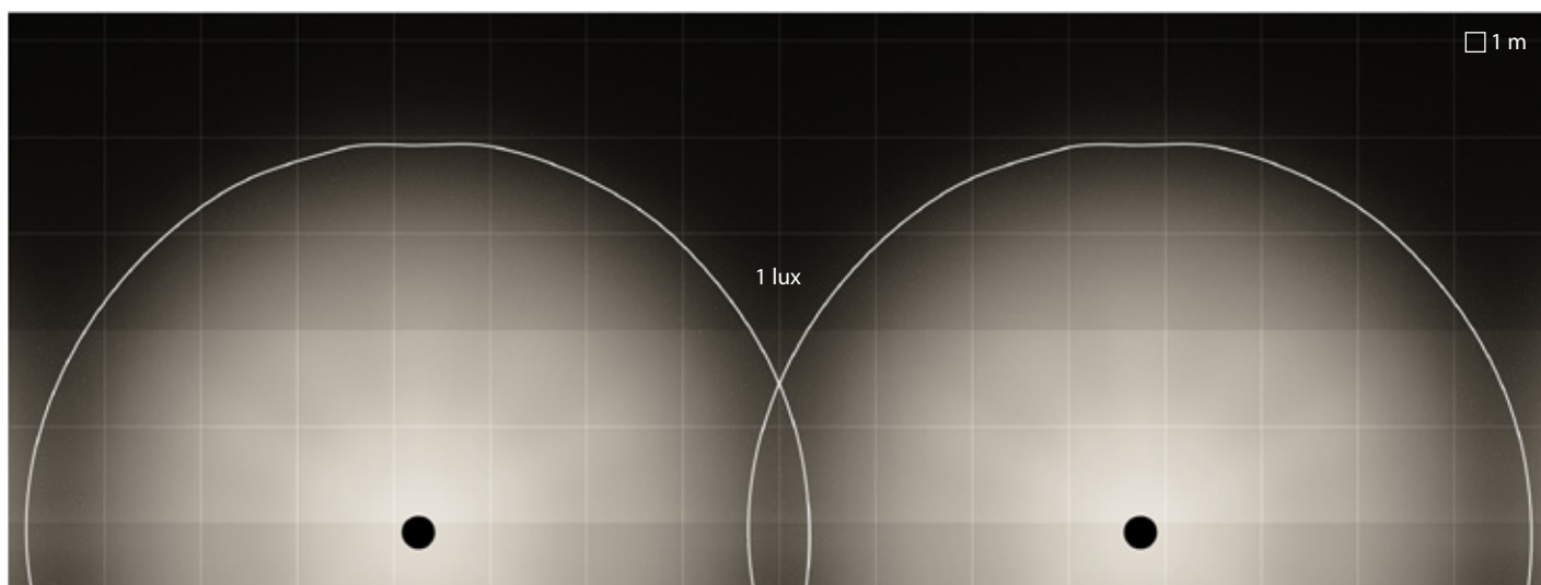
SPILLO MINI | C/EW | linéaire
