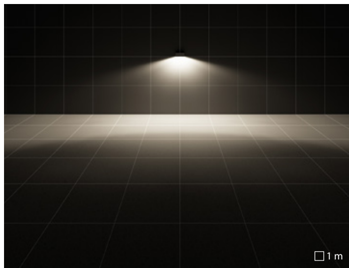
MIMIK 30 | CP/T2 optique pour velos et pietons type 2
