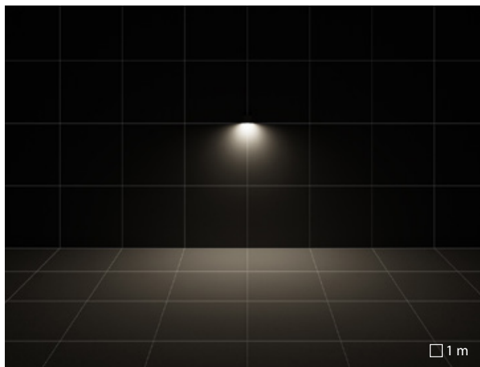
MIMIK 10 FLAT M | A/W optique asymétrique diffusante
