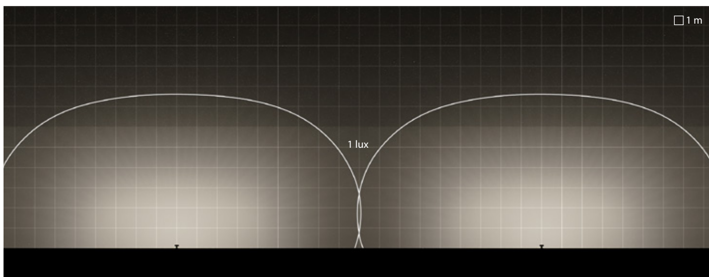
AMON WALL | A30/M | linéaire
