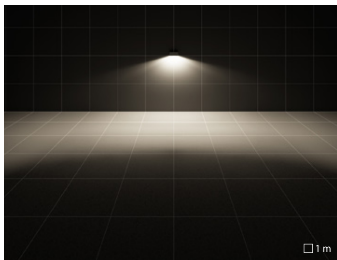
MIMIK 30 | CP/T3 optique pour velos et pietons type 3
