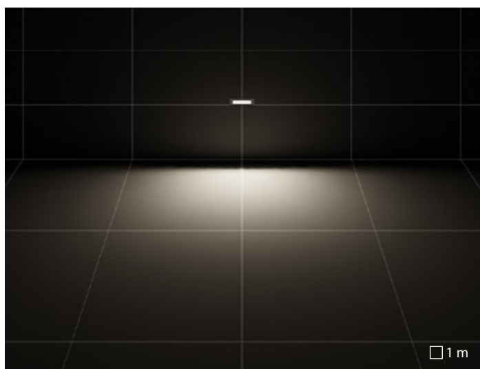
A37/M optique asymétrique moyenne
