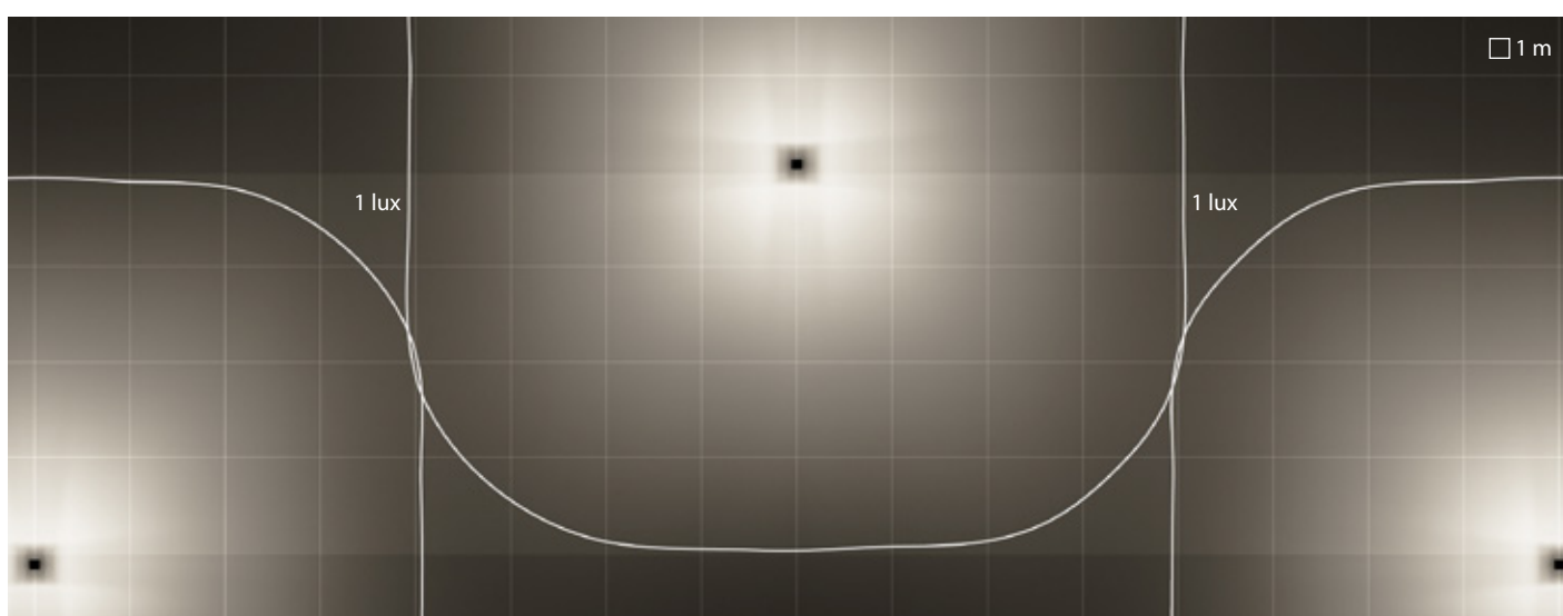
S/W optique symétrique diffusante
