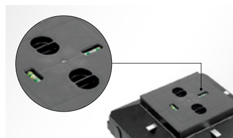
Tous les boîtiers d'encastrement STEEL SQUARE sont dotés d'un couvercle contenant des bulles de niveau pour faciliter leur mise en place correcte en phase d'installation.
