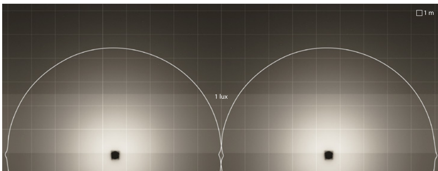
KHA 9 | C/EW optique circulaire extra diffusante
