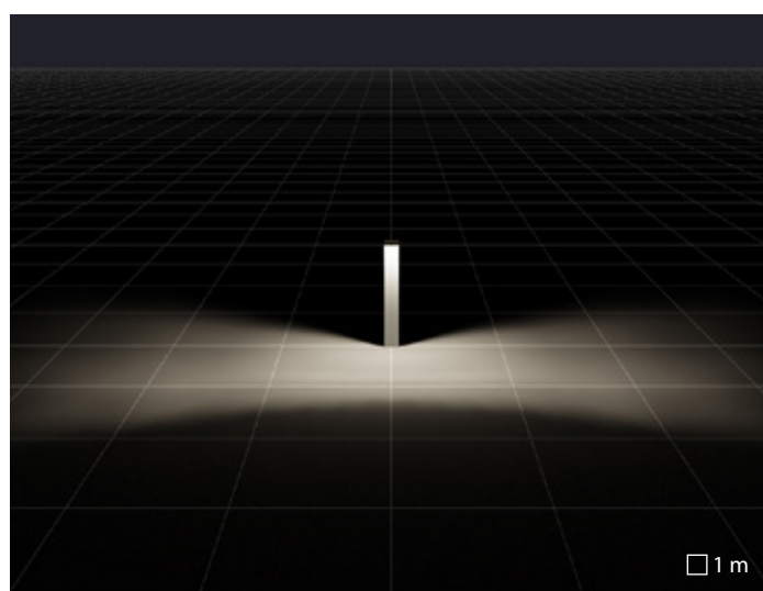
MIMIK 10 POST 1000 | CP/T3 optique pour velos et pietons type 3
