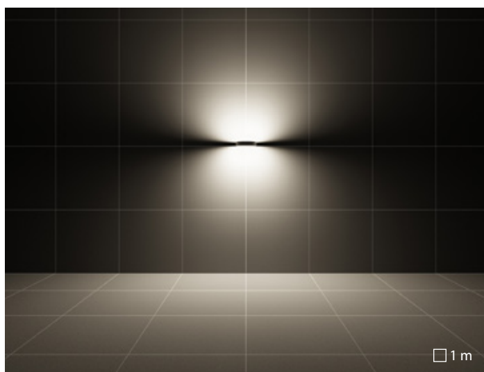
MASK+ B | S/EW optique symétrique extra diffusante
