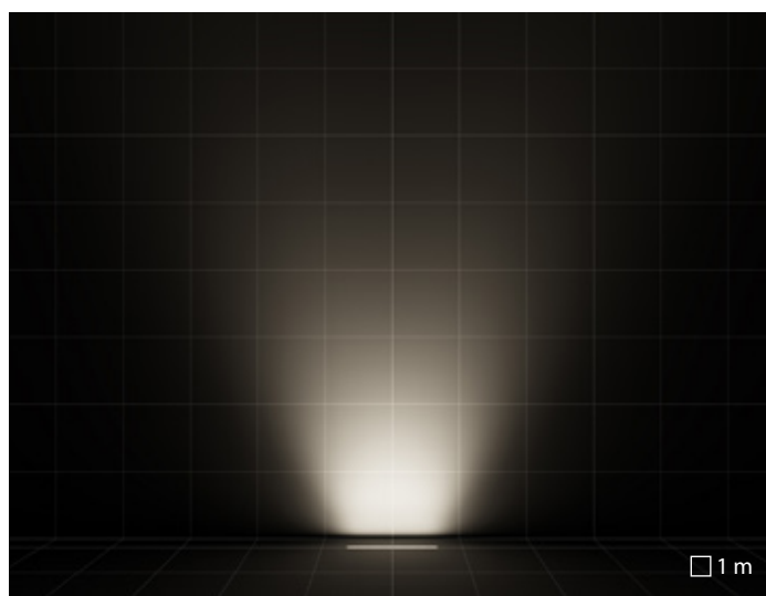
ELL 40°x60° optique elliptique
