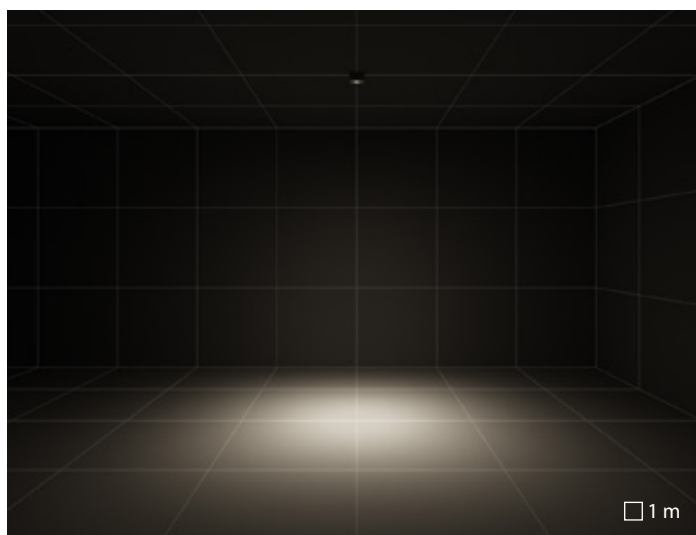
MIMIK 10 CEILING | C/I optique circulaire intensive
