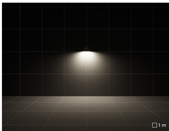
MASK+ M | S/EW optique symétrique extra diffusante
