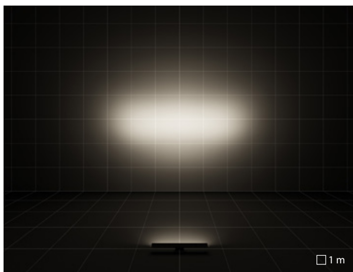
ELL 15°x45° optique elliptique
