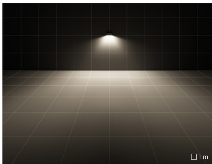
MIMIK 30 | A60/W optique asymétrique diffusante
