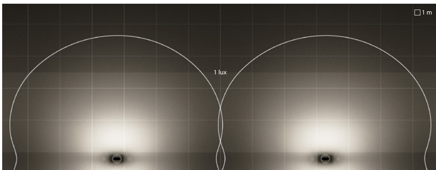
AMON MINI | SOFT S/EW | linéaire
