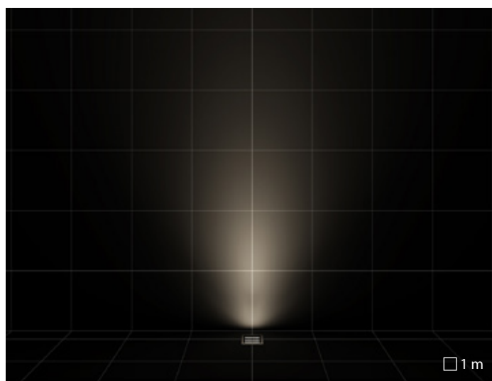
ELL optique elliptique
