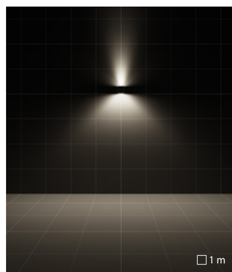
A15/M asymmetrische mittlere Optik + S/I symmetrische Optik gebündelt
