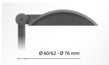
Versionen KYRO+ 2 sind geeignet für Montage an Masten mit Ø 60/62 - Ø 76 mm
